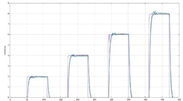
Abbildung 4a: Test von 4 Sensorsystemen zeitgleich mit 2, 4, 6 und 8 Vol.-% H 2 in 13 Vol.-% O 2 . Gemessen mit einem Gesamtflow von 2.000 sccm.
